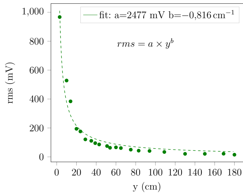
FIGURE 1 – Evolution de la valeur efficace aux bornes d'un micro en fonction de sa distance y à l'émetteur.
